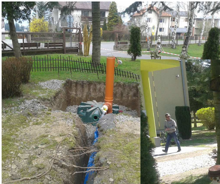
Umelý vodný tok s fontánou a podzemným zásobníkom na dažďovú vodu s čerpadlom
