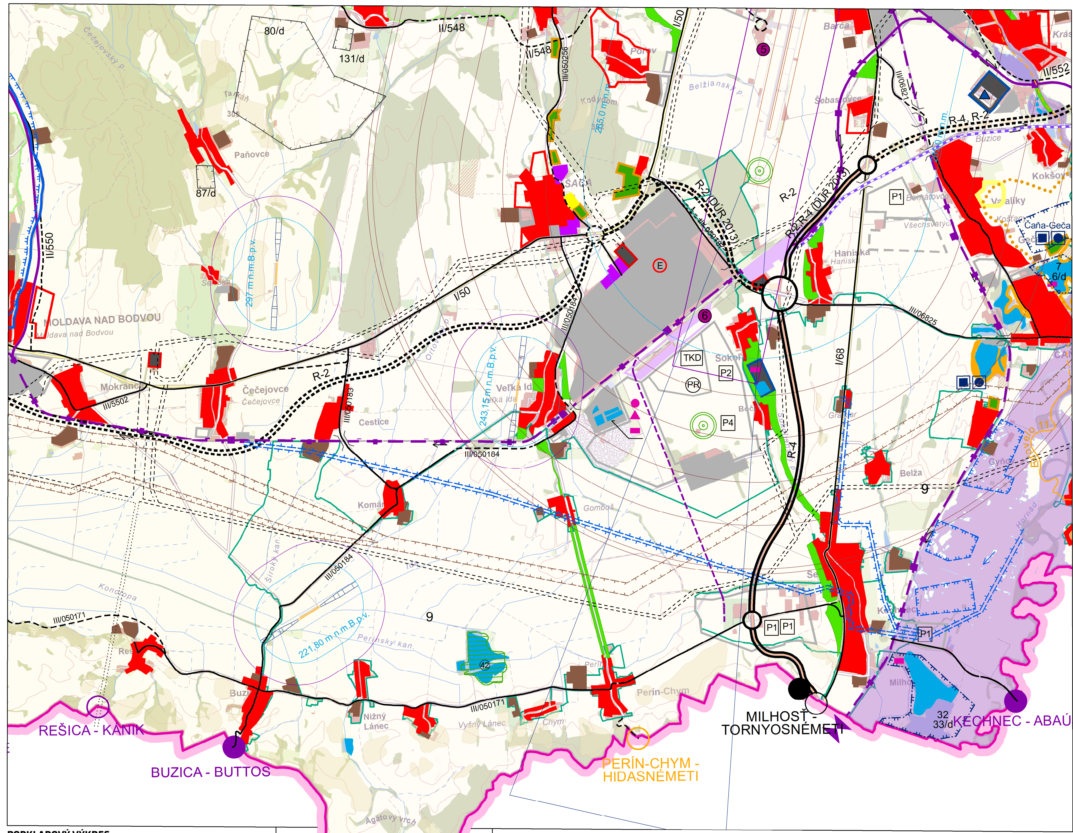
PODKLADOVÝ VÝKRES
